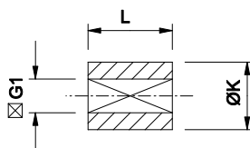
Manchon d'accouplement standard fourni avec l'appareil
