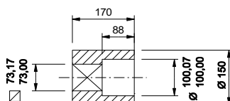
Manchon d'accouplement standard fourni avec l'appareil
