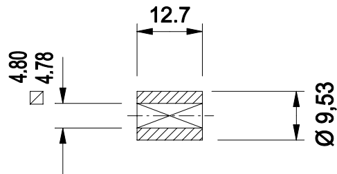
Manchon d'accouplement (fourni avec l'actionneur)
